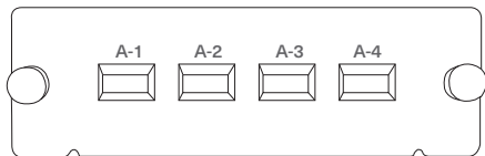
FHD-4MTPMESHSMF/HD-4MTPMESHOM4
